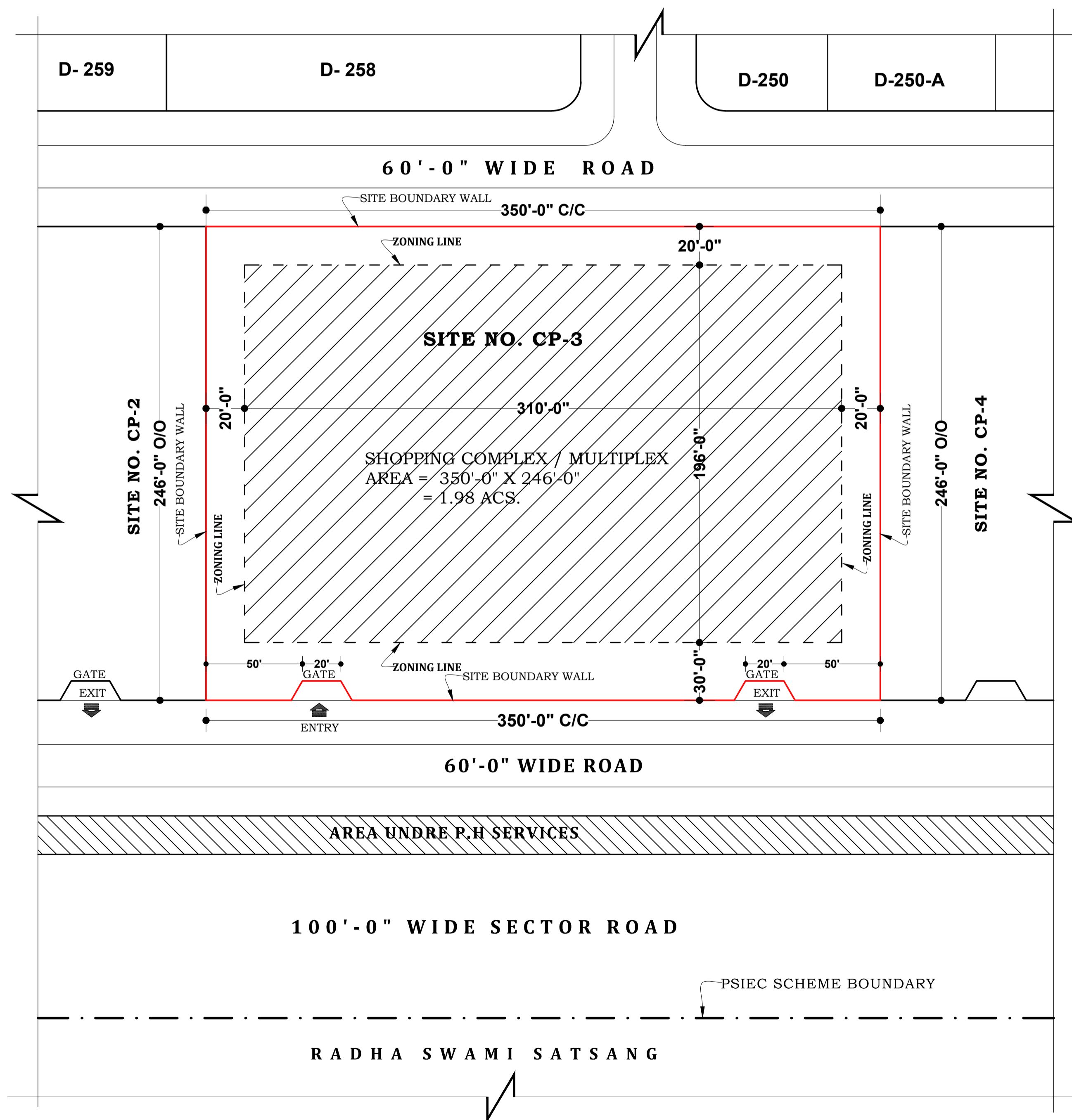
KEY PLAN (NO. TO SCALE)
